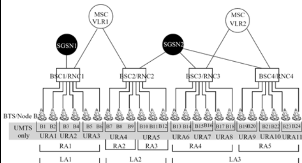
Fig. 2.3 LAs, RAs, and URAs
