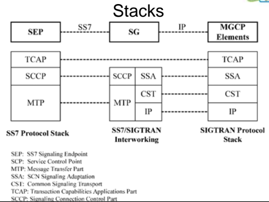
Fig 10.3 TCAP-SIGTRAN Protocol
