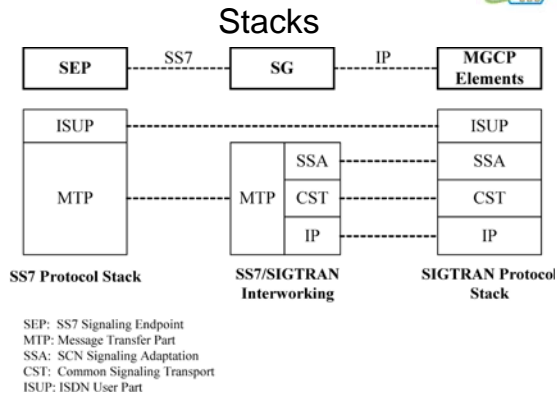
Fig. 10.2 ISUP-SIGTRAN Protocol
