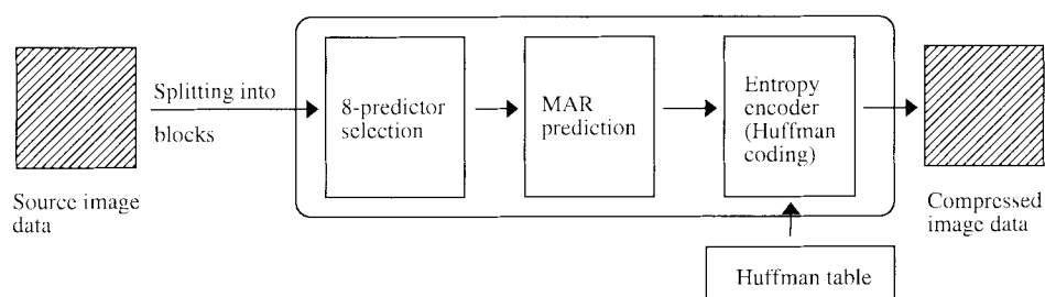
Fig. 3. Encoder of the APMAR.
